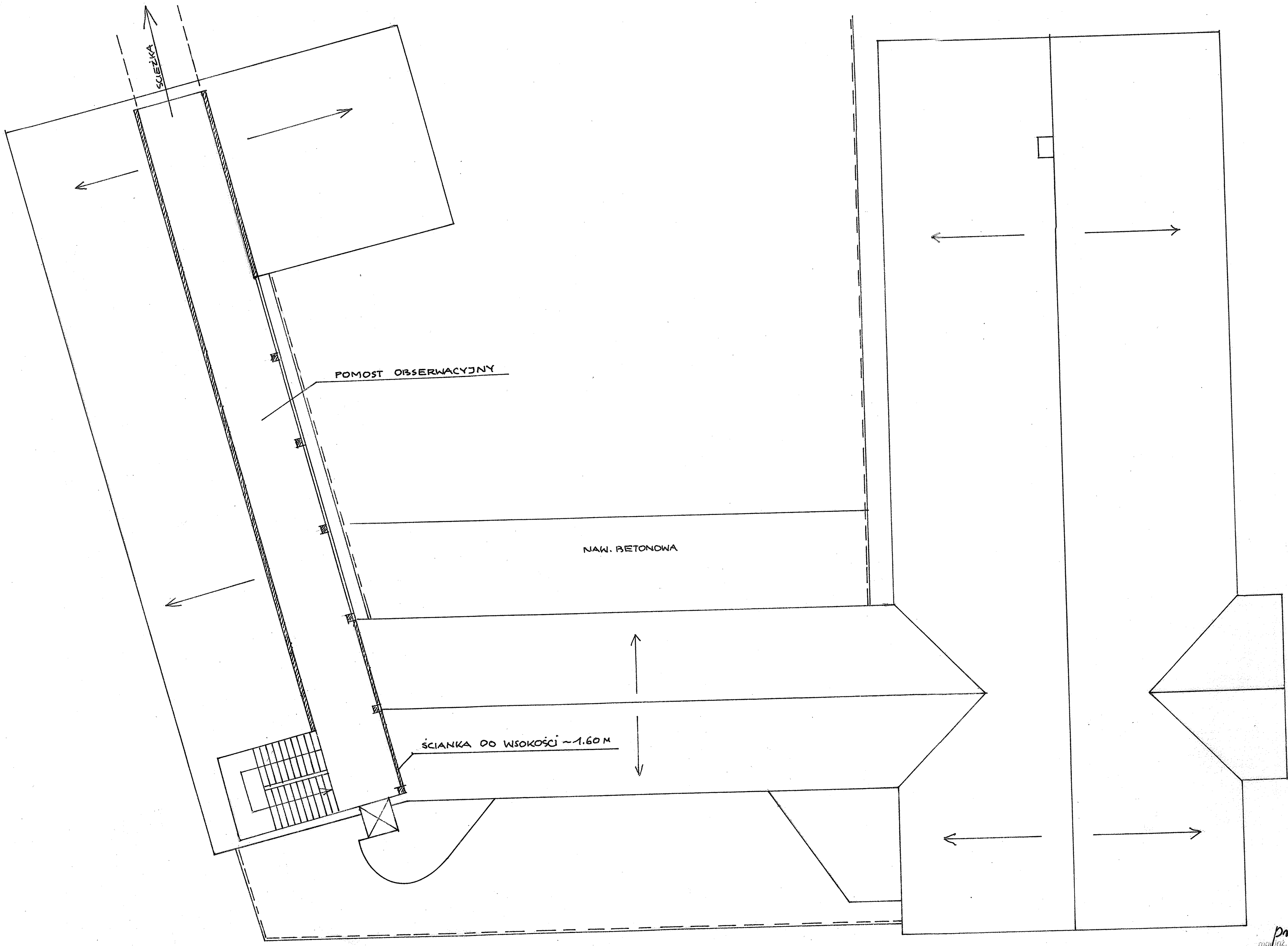
RZUT POŁĄCI DACHOWYCH I POMOSTU OBSERWACYJNEGO 1 : 100
